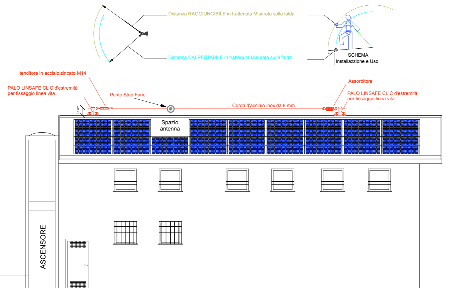
PROSPETTO OVEST
